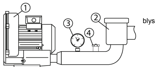
Pav. nr. 5: Oro siurblys su priedais
